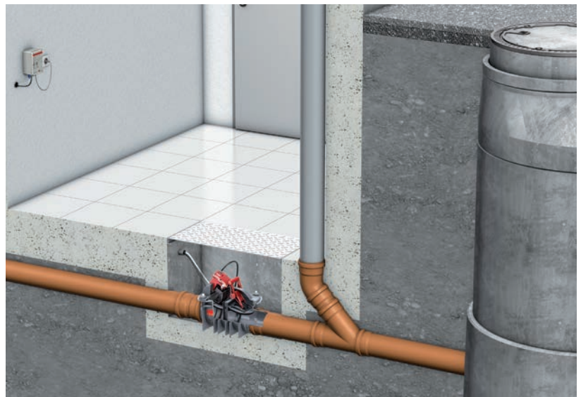
Rückstausicherung – bei Gefälle zum Kanal
