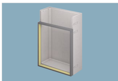
Betonlichtschacht in druckwasserdichter Ausführung mit umlaufend aufgebrachten Dämmrahmen zum Aufstellen einer Hinterfüllplatte und zusätzlichem Befestigungsbereich zur Verschraubung der Hinterfüllplatte mit dem Schacht
