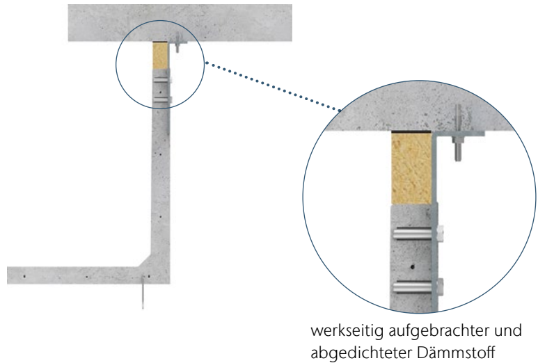
DWD-Montage auf Dämmung
