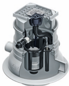
Unterflurhebeanlage Multi-UF
