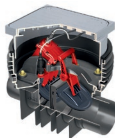
Rückstauautomat Quatrix
