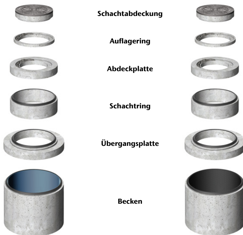
Beispielhafter Schachtaufbau Fettabscheider beschichtet
