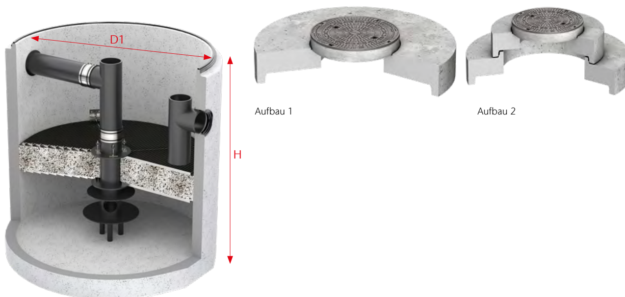
Filtrationsschacht Typ 2200
