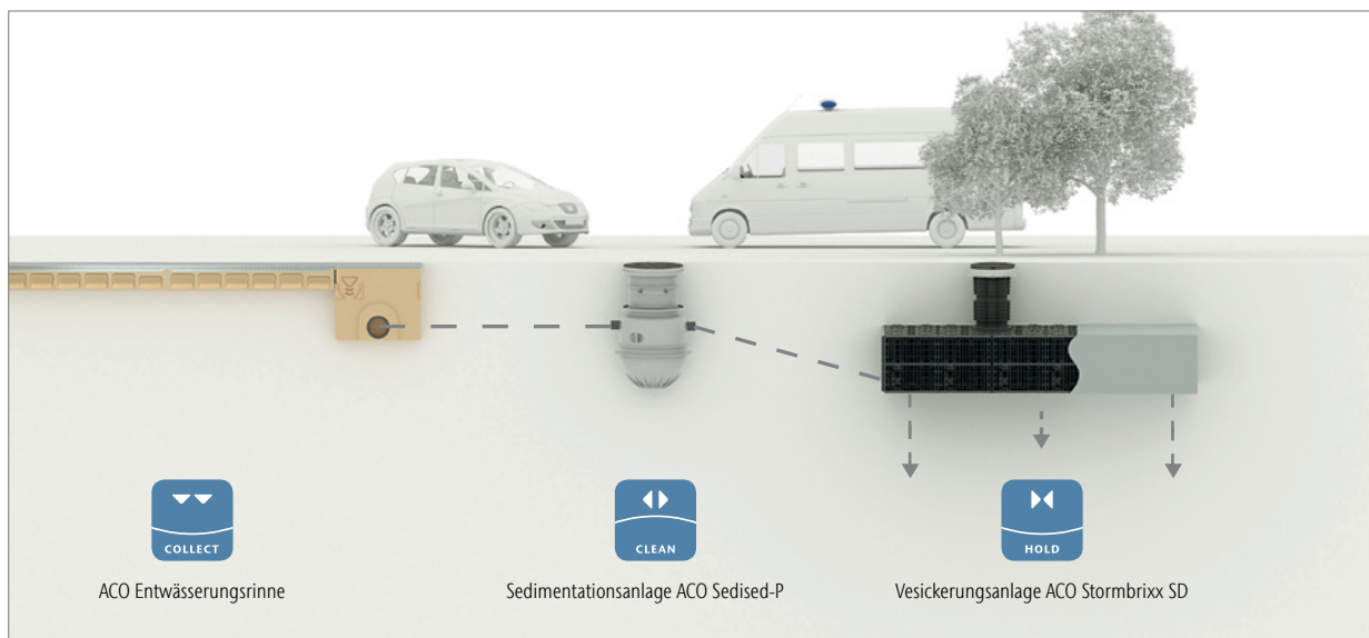
ACO WaterCycle für eine Regenwasserversickerung mit ACO Stormbrixx
