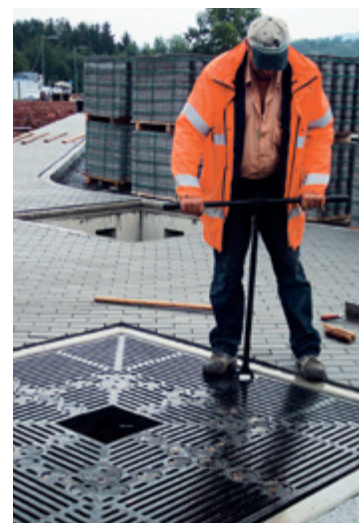
Teilroste werden tragfest verbunden
