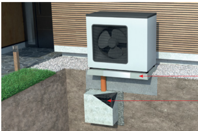
Wärmepumpenfundament
