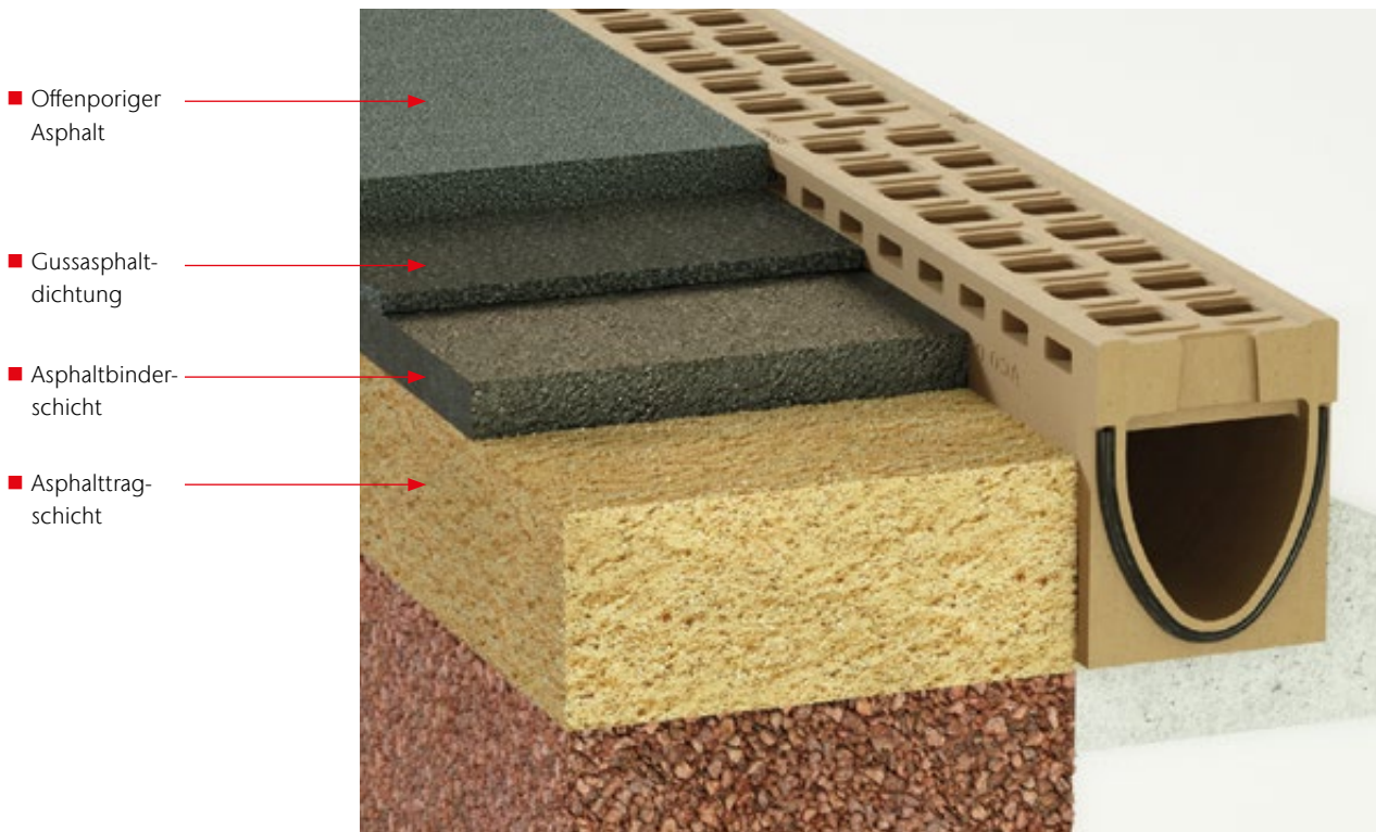
Schichtenaufbau
