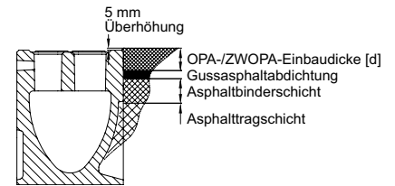
Beispielhafter Schichtenaufbau
