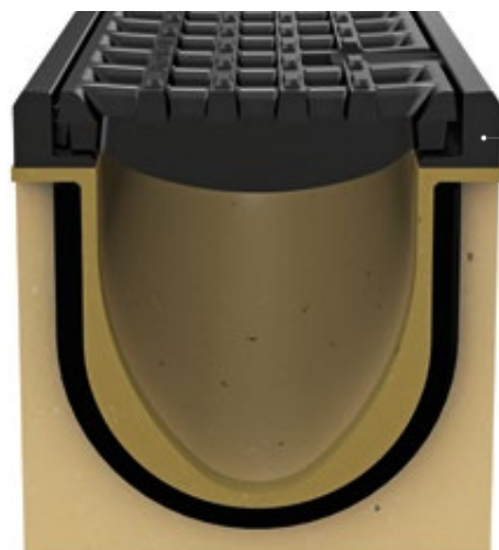
Starke Gusszarge
