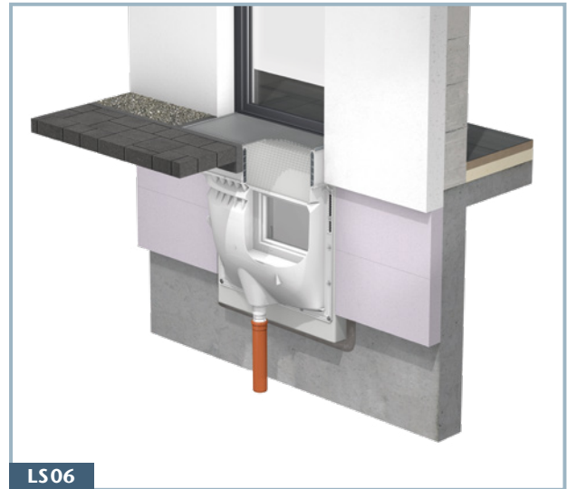
Barrierefreier Übergang – Lichtschacht vor Terrassentür S. 50–57
