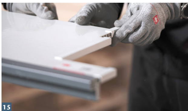
15 Abschnitte der Wandanschlussprofile auf Schnittflächen stecken.
