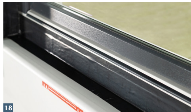
Abdichtung zur Terrassentür z.B. mit KSK-Bahn oder Aqua Blocker herstellen. Kondensatöffnung ggf. aussparen.
