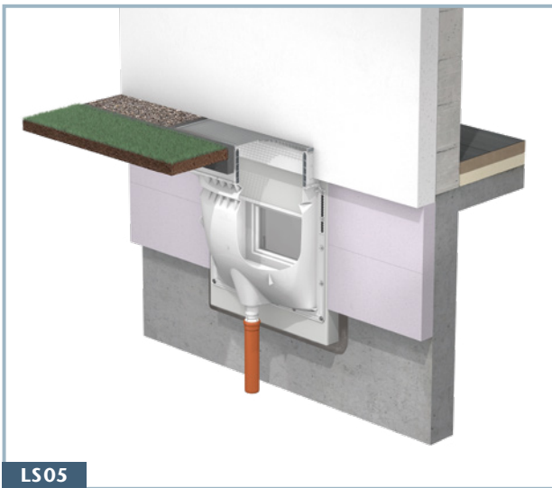
Sauberer Übergang – Lichtschacht zum vorspringenden WDVS mit fixem Aufstockelement S. 42–49
