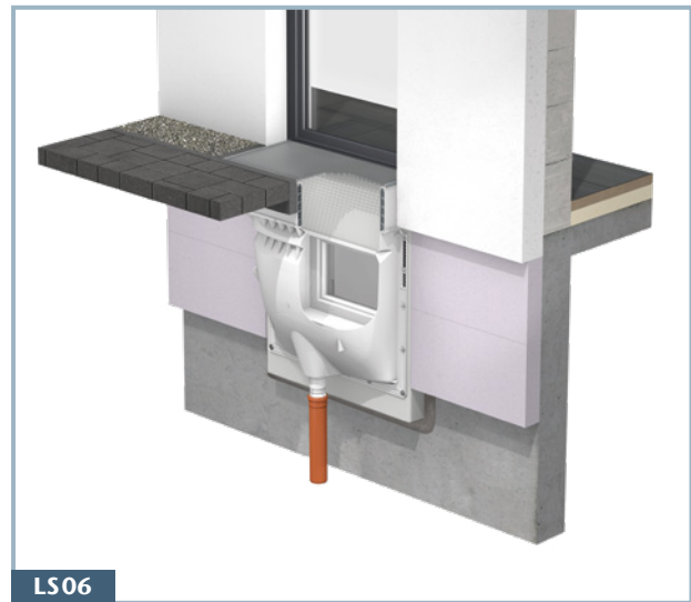
Barrierefreier Übergang – Lichtschacht vor Terrassentür S. 50–57
