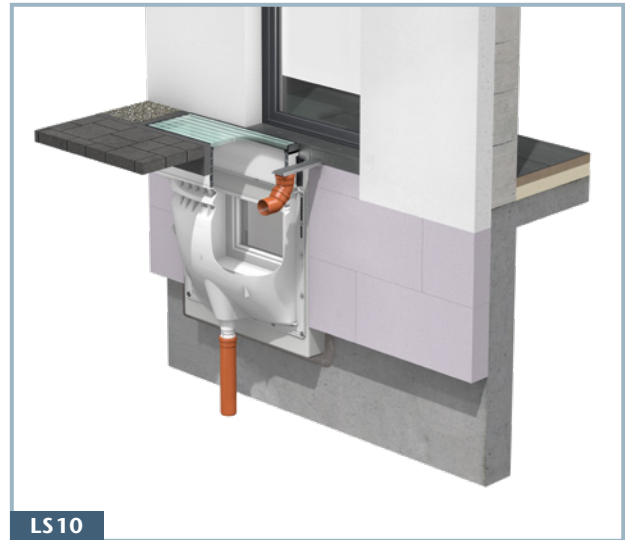
Barrierefreier Übergang – Lichtschacht mit Glasabdeckung dezentral vor Terrassentür S. 82–89
