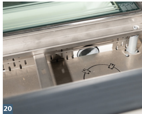
20 Rinnenentwässerung durch Aufstockelement hindurch herstellen.
