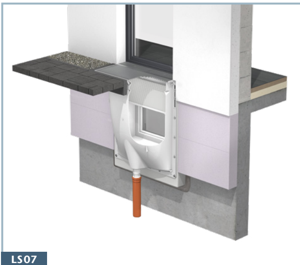
Barrierefreier Übergang – Lichtschacht und Fassadenrinne vor Terrassentür S. 58–65
