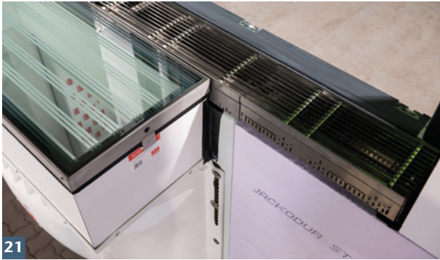
... Anpassung der ACO Fassadenrinne.
