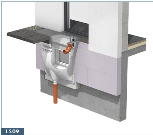
Barrierefreier Übergang – Lichtschacht mit 4-seitigem Aufstockelement dezentral vor Terrassentür S. 74–81
