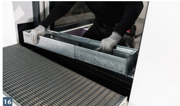
Baulängen-Anpassung und Montage der ACO Profiline Fassadenrinne.
