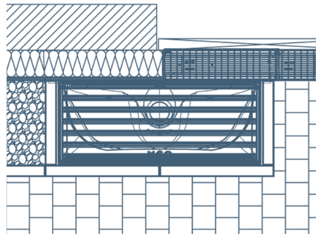
Anschluss der Fassadenrinne mittels eines Leibungsablaufelements an die Entwässerung.
