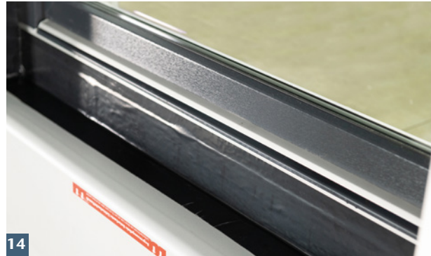
ACO Therm® Block z.B. mittels KSK-Bahn oder Aqua Blocker vor Hinterläufigkeit schützen. Abdichtung zur Terrassentür z.B. mit KSK-Bahn oder Aqua Blocker herstellen. Kondensatöffnung ggf. aussparen.
