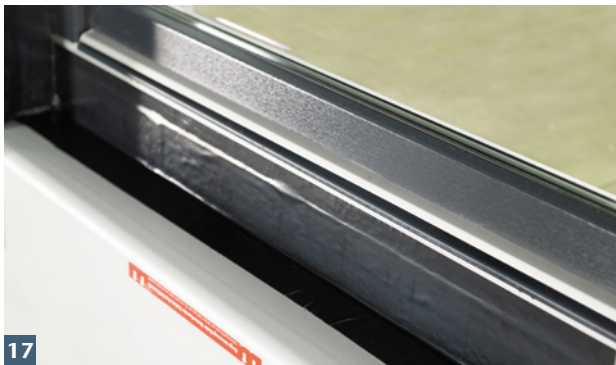
Abdichtung zur Terrassentür z.B. mit KSK-Bahn oder Aqua Blocker herstellen. Kondensatöffnung ggf. aussparen.
