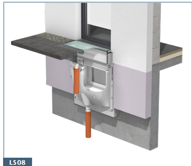
Barrierefreier Übergang – Lichtschacht mit belüfteter Glasabdeckung vor Terrassentür S. 66–73
