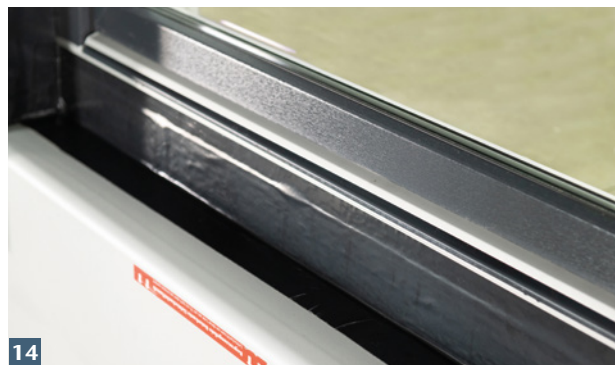
14 Abdichtung zur Terrassentür z.B. mit KSK-Bahn oder Aqua Blocker herstellen. Kondensatöffnung ggf. aussparen.
