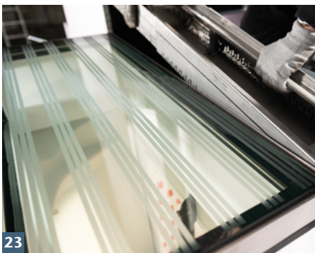
ACO Fassadenrinne anpassen und montieren.
