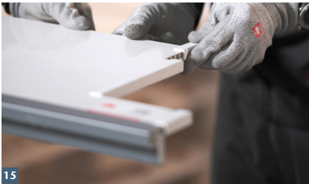
Abschnitte der Wandanschlussprofile auf Schnittflächen stecken.
