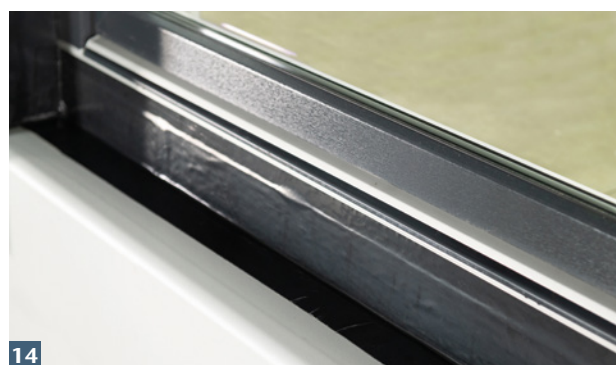
14 ACO Therm® Block z.B. mittels KSK-Bahn oder Aqua Blocker vor Hinterläufigkeit schützen. Kondensatöffnung ggf. aussparen.
