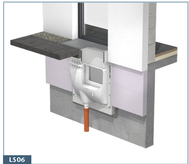
Barrierefreier Übergang – Lichtschacht vor Terrassentür S. 50–57
