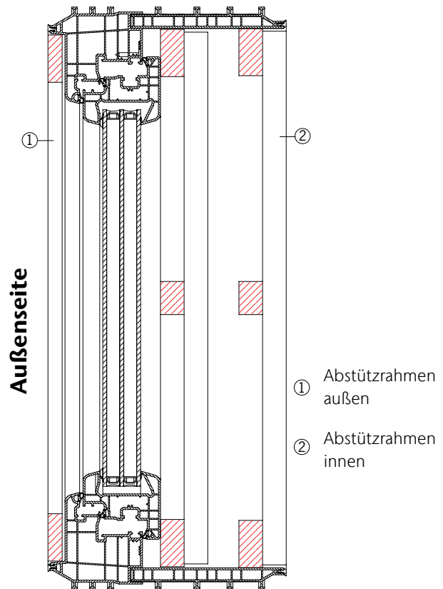
Schnitt senkrecht
