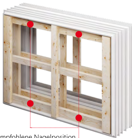
Empfohlene Nagelposition für äußere Befestigung
