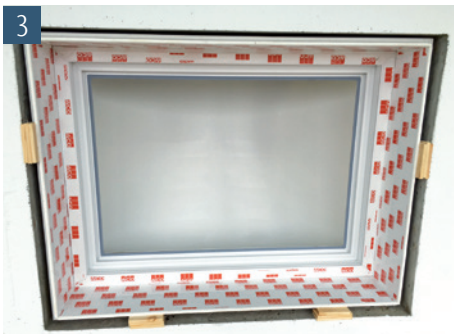
3 Leibungselement ausrichten und verklotzen
