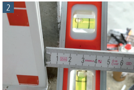
2 1 cm Abstand umlaufend zur Innenwand einhalten
