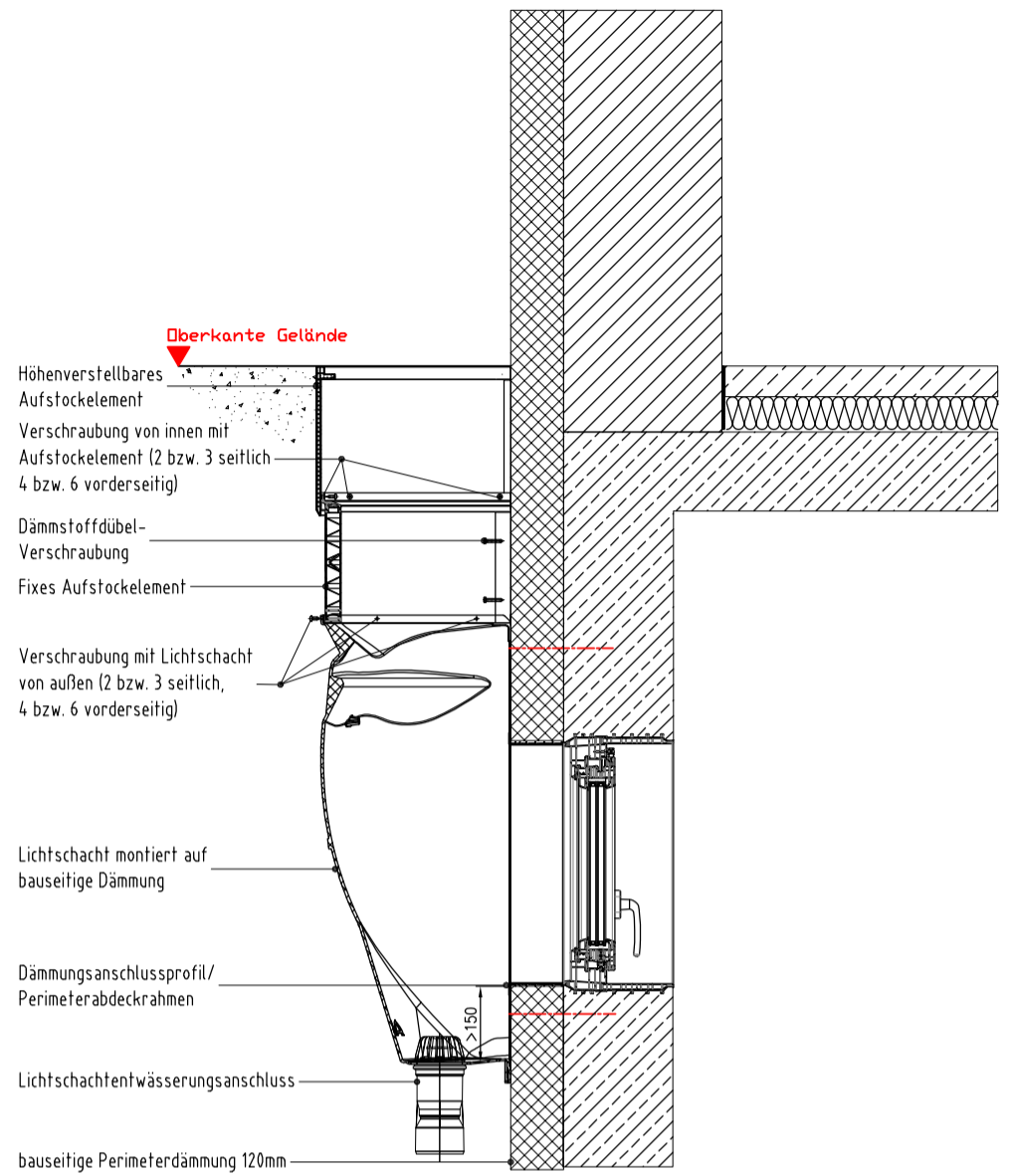
1 höhenverstellbares und 1 fixes Aufstockelement - begehbar - Montage auf Perimeterdämmung -
